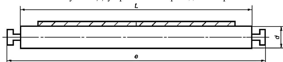
Рисунок 5 Одно-роликовая опора
