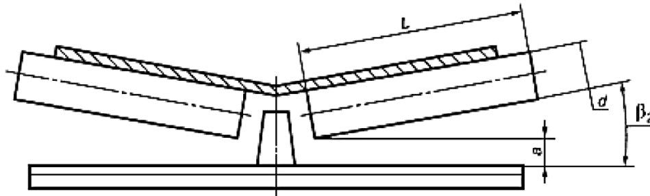
Рисунок 3 Жесткая двух-роликовая опора 180^\circ - 2\beta_2
