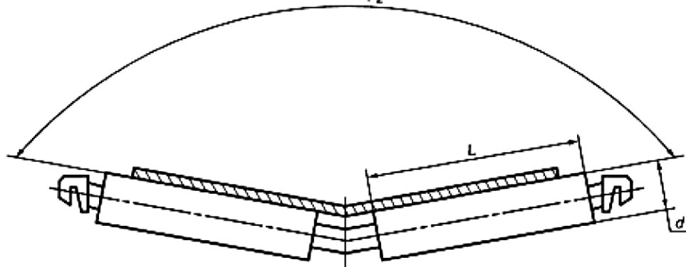
Рисунок 4 Двух-роликовая гирляндная опора
